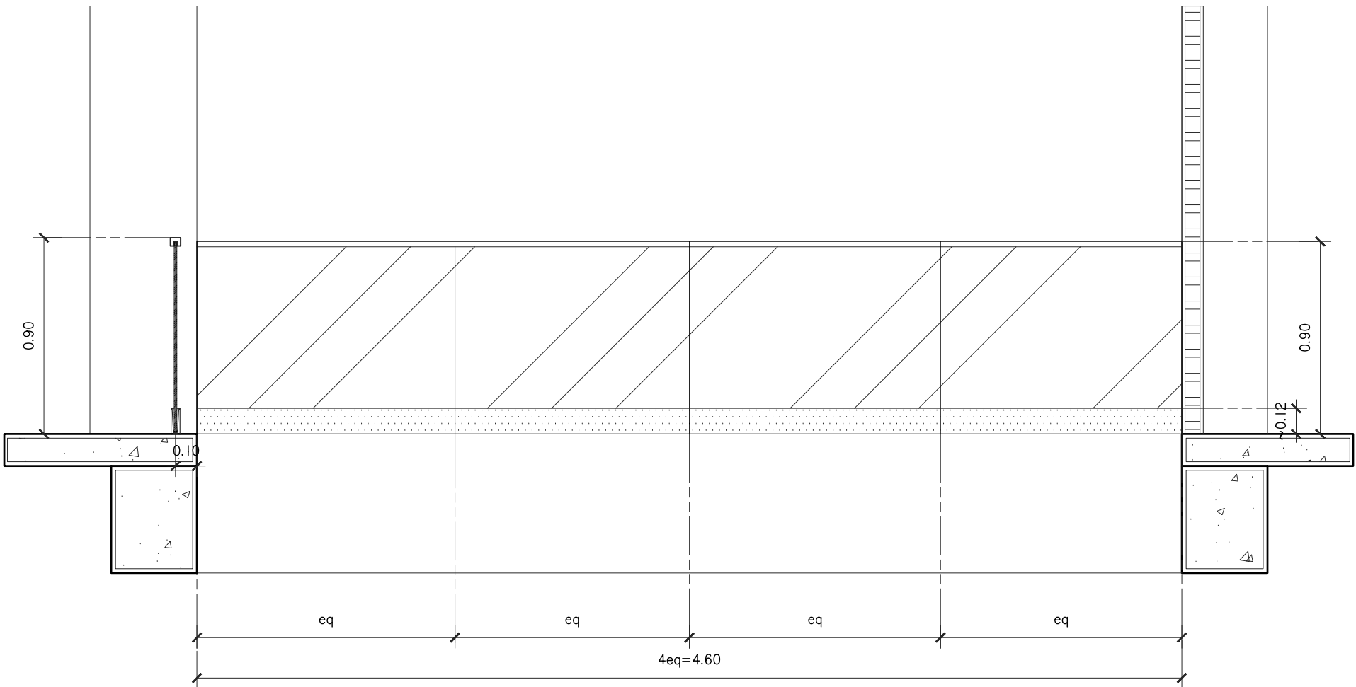
รูปด้าน B มาตราส่วน 1 : 25
