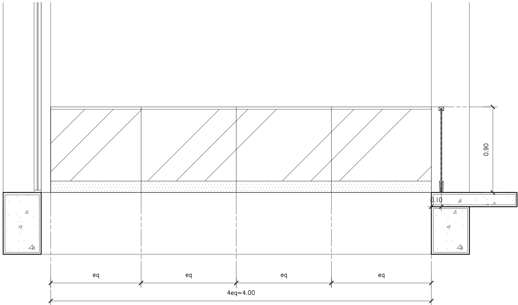
รูปด้าน A มาตราส่วน 1 : 25
