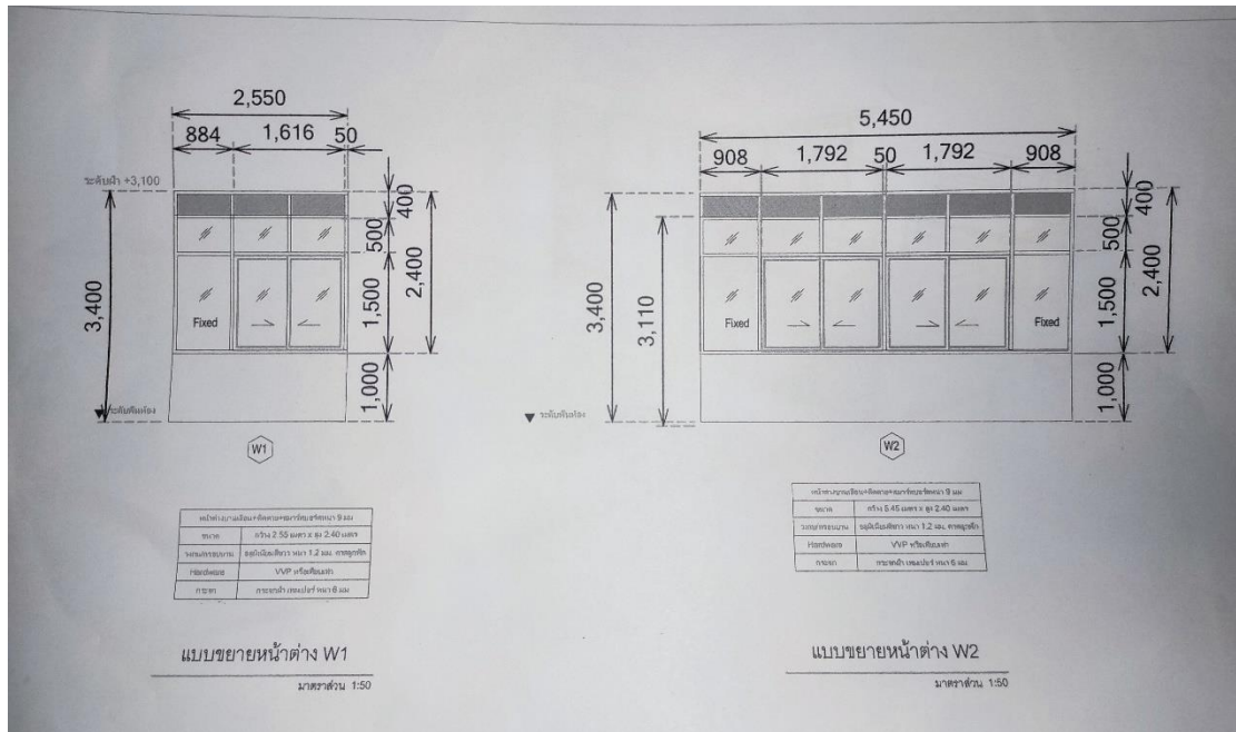
รูปประกอบ 4 รูปแบบรายละเอียดหน้าต่าง W1 และ W2
