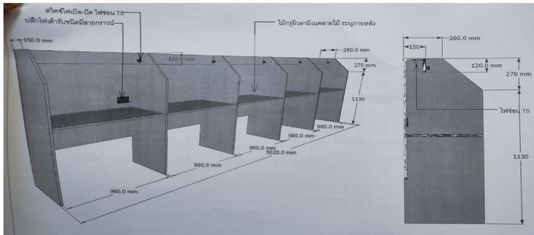
รูปประกอบ 3 รูปแบบรายละเอียดโต๊ะอ่านหนังสือ
